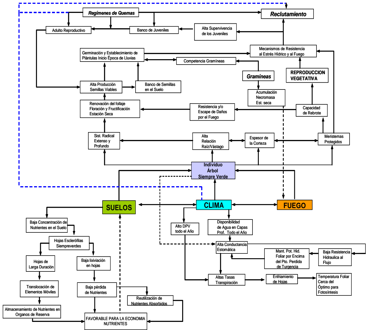
Figura 1. Esquematación de los principales factores, procesos y sus interacciones, que influyen en la ecología de la regeneración de las leñosas siempreverdes de las sabanas estacionales.
